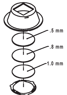
Optional Filter Kit - IK163 P/N 7576 可选 过滤套件 - IK163 P/N 7576
